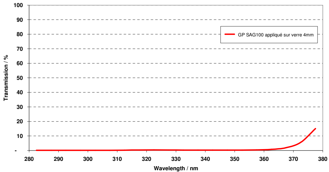
GP SAG 100 : Transmission UV suivant EN410 (mesuré sur Cary 5000)
